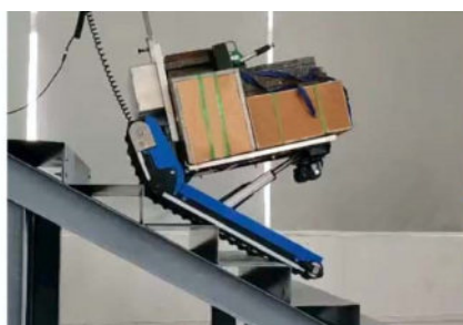
DME400 in uso
